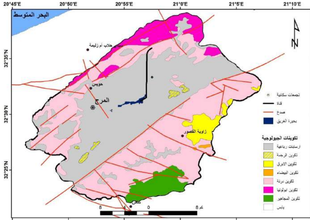
شكل 2: الخارطة الجيولوجية لحوض سهل المرج، المصدر: الخارطة الجيولوجية، لوحة بنغازي، (رولبخ، 1974)
